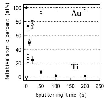
Fig. 1 金蒸着Ti板上のAu, Tiのat%
